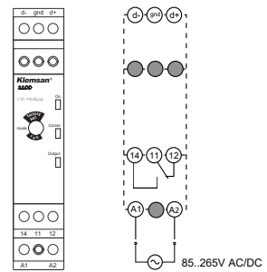
KR I/O 1100
