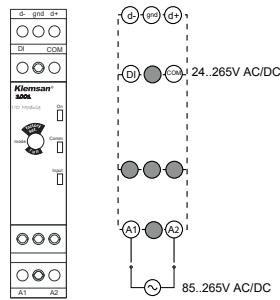
KR I/O 1001
