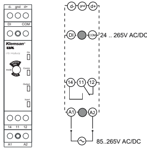
KR I/O 1101
