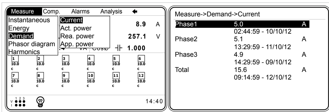
Fig. 3-80 Current Menu
